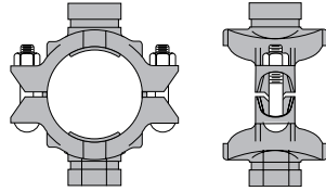
Fig. 7048 — Groove x Groove
