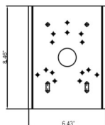
VT-TPLMT Universal Pole Mount Adapter (VT-TWM03X or VT-TWMT-A2 + VT-TJB010 Req)
