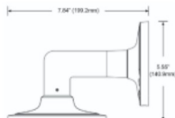
VT-TWMT-A2 Wall Mount (VT-TJB010 Req)
