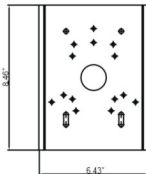
VT-TPLMT Universal Pole Mount Adapter [VT-TWM03X or VT-TWMT-A2 + VT-TJB010 Req]
