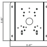
VT-TCNMT Universal Corner Mount Adapter [VT-TWM03X or VT-TWMT-A2 + VT-TJB010 Req]
