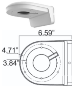
VT-TWMT-4 Optional Wall Mount
