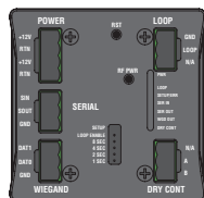
Module d'interface Wiegand S2W-001
