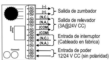
Fig. 10 – Vista superior de temporizador
