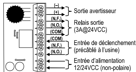
Fig. 10 – Vue de dessus de module minuterie
