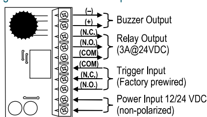
Fig. 10 – Timer Module Top View
