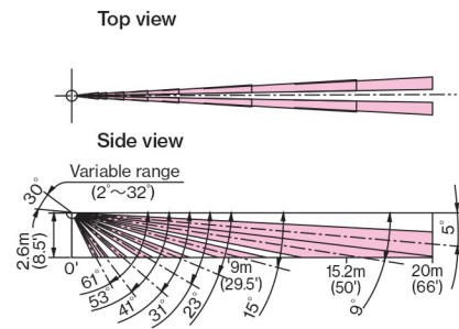
PA-6820E (Vertical curtain)
