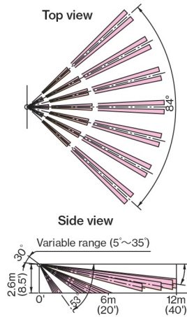
PA-6820E (Vertical curtain)
