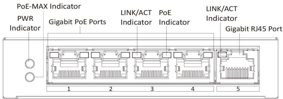
DS-3E0505P-E
