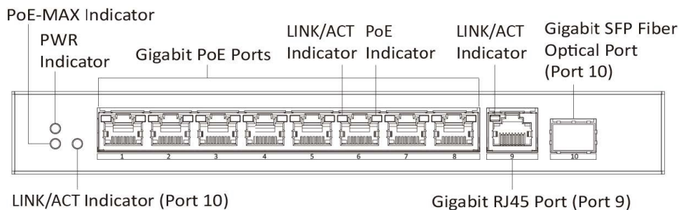
DS-3E0510P-E
