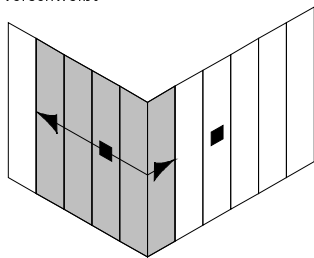
Eckverbindung Wand/Wand durchgehend verschweißt
