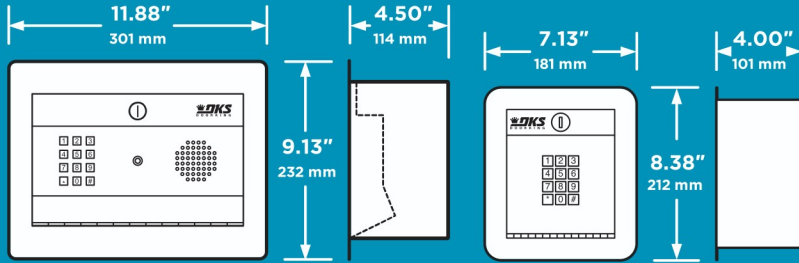
1504 Flush
