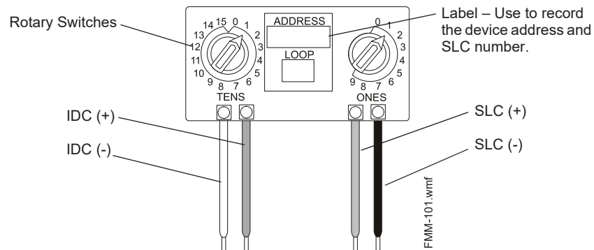
Figure 5.8 SK-MINIMON Mini Monitor Module
