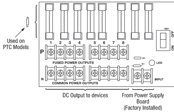
Fig. 4 - PD16W/PD16WCB
