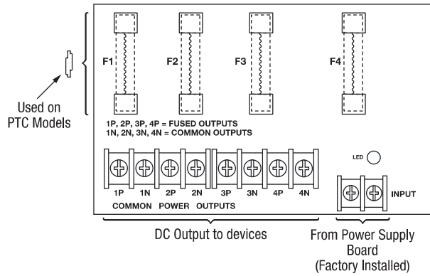
Fig. 2 - PD4/PD4CB
