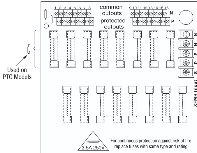
Fig. 4 - PD16W/PD16WCB
