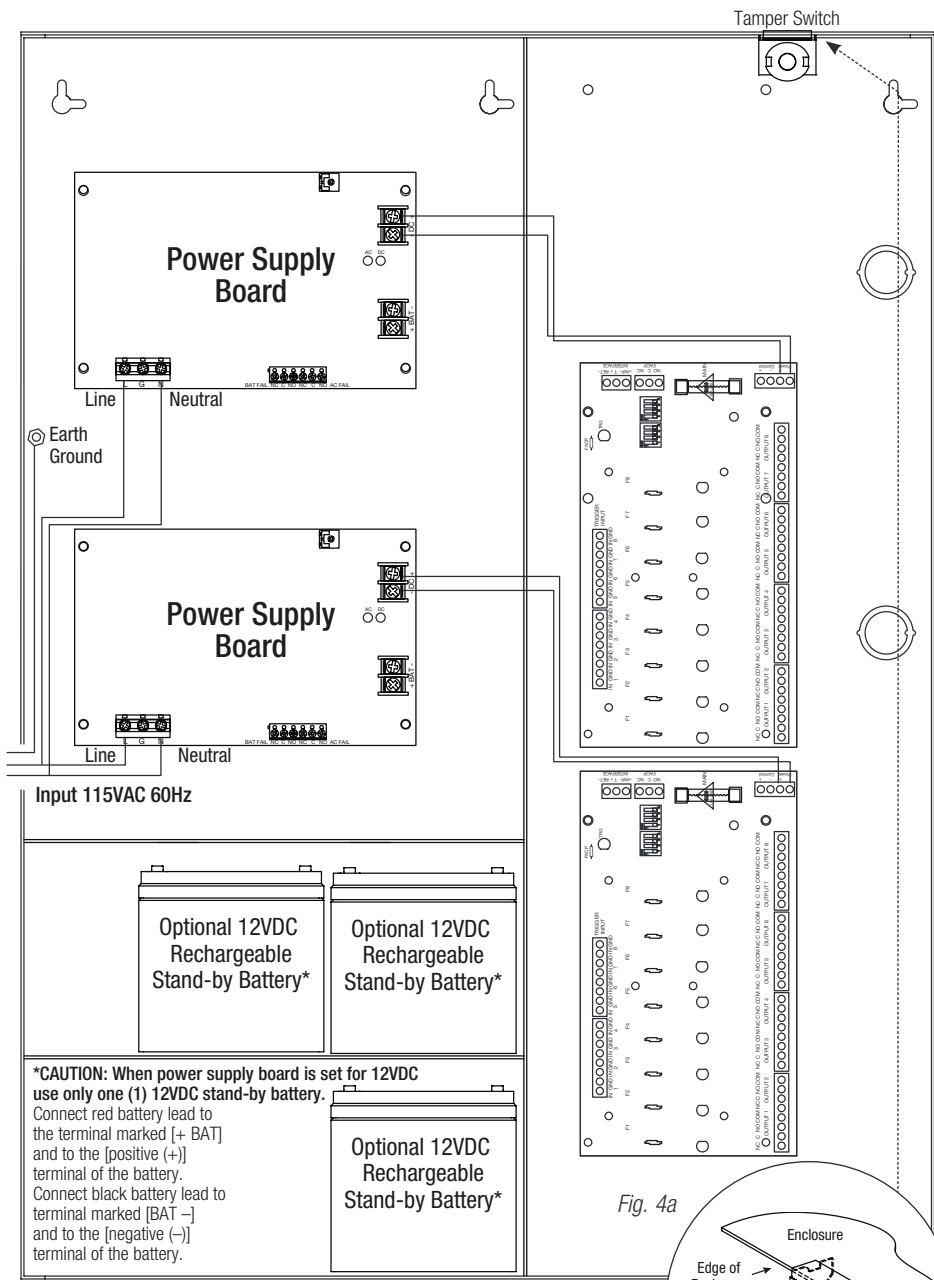
Fig. 4 - Maximal75D
