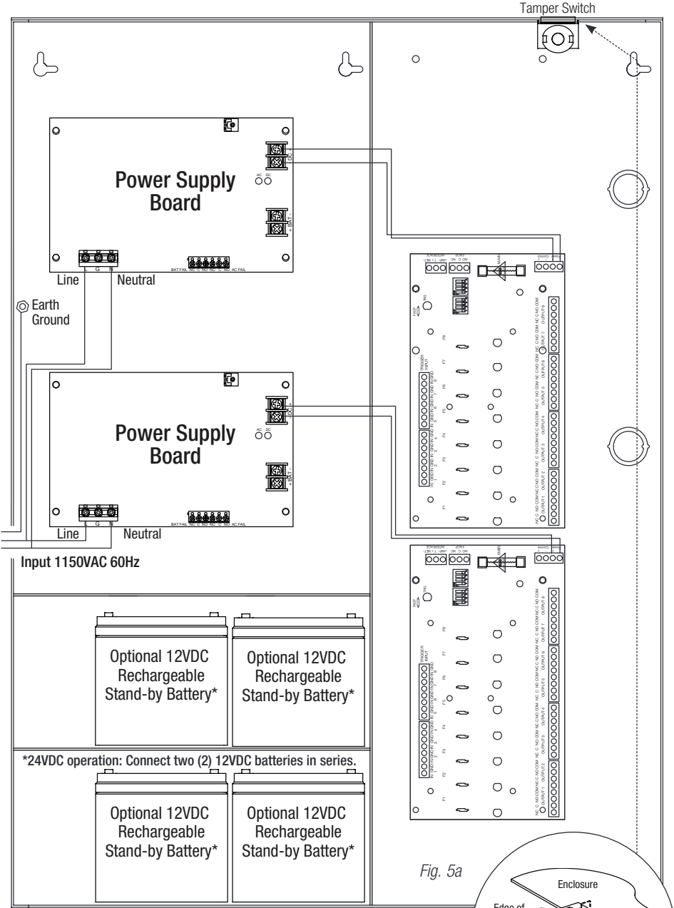
Fig. 5 - Maximal77D
