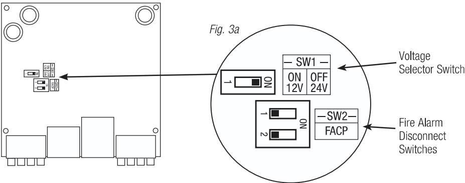
Fig. 3 - Entrada2DMT PC Board
