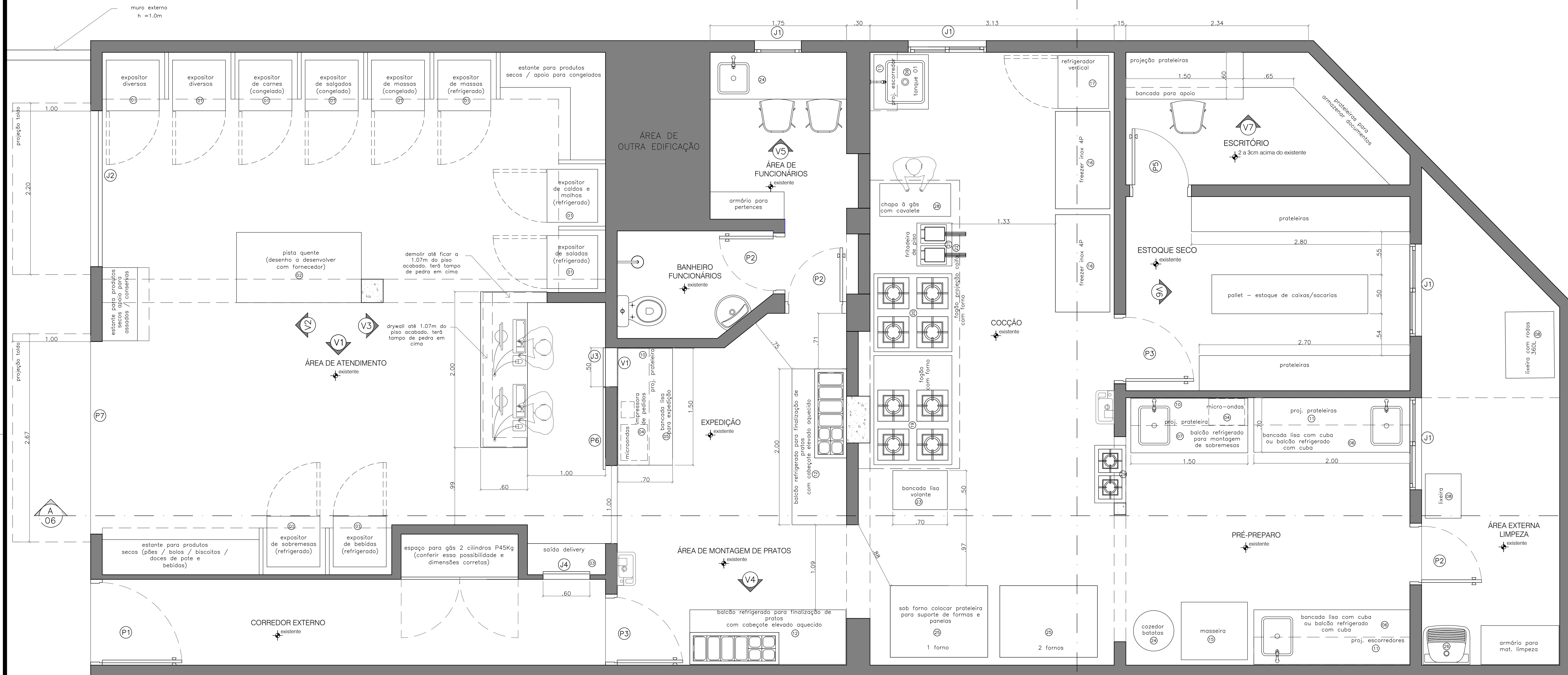
PLANTA DE LAYOUT ESCALA 1:25
