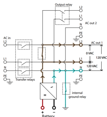
Vermogenstroom: omvormer-modus
