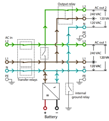
Vermogenstroom, gesplitste fase invoer
