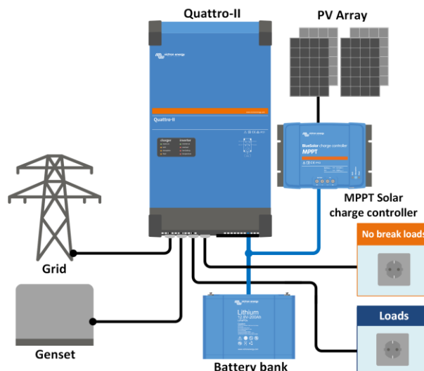
Toepassing met MPPT-PV-laadregelaar
