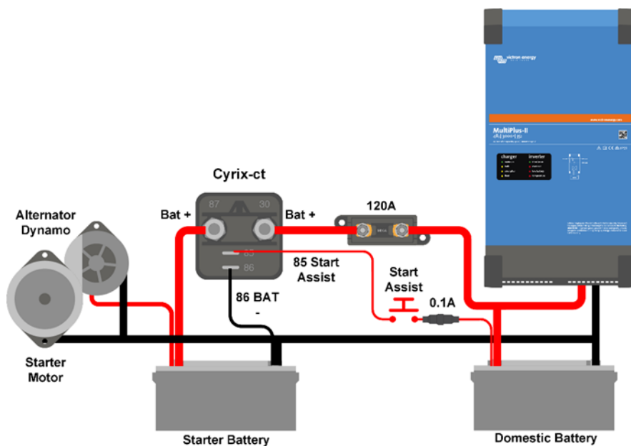
Cyrix-ct 12/24-120: aansluitschema
