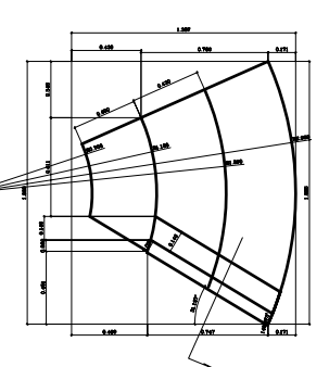
Ashler NM18C plan 1:50
