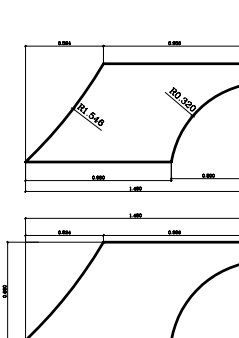
NM19A Section 1:50
