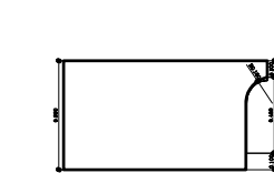
NM11-A Section-A 1:50
