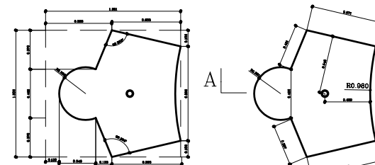
NM11-A Base Plan 1:50
