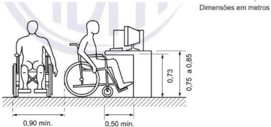
Figura 152 – Terminais de consulta – Exemplo – Vista lateral
