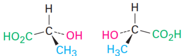
Enantiomers
