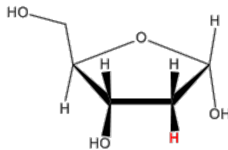
Deoxyribose
